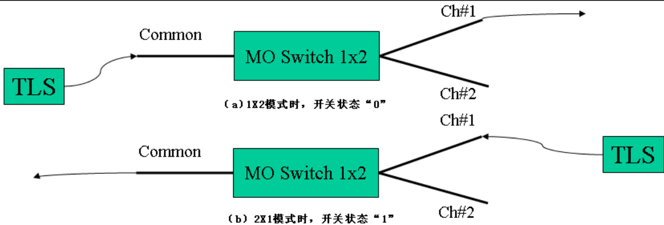
图 6. 2x1 光开关
