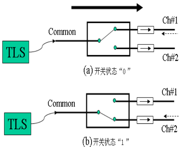
图 4 1x2 模式
