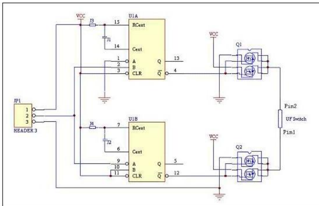
图 3. 驱动电路图
