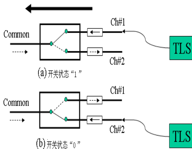
图 5 2x1 模式
