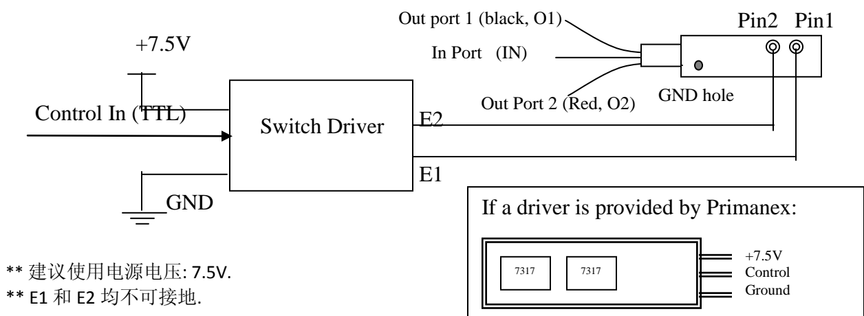
图 2. 1X2 光开关与驱动电路的连接图
